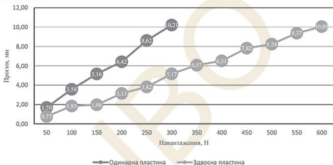
Рис. 5. Графік зміни середніх величин прогину одинарних і здвоєних пластин залежно від величини навантаження
